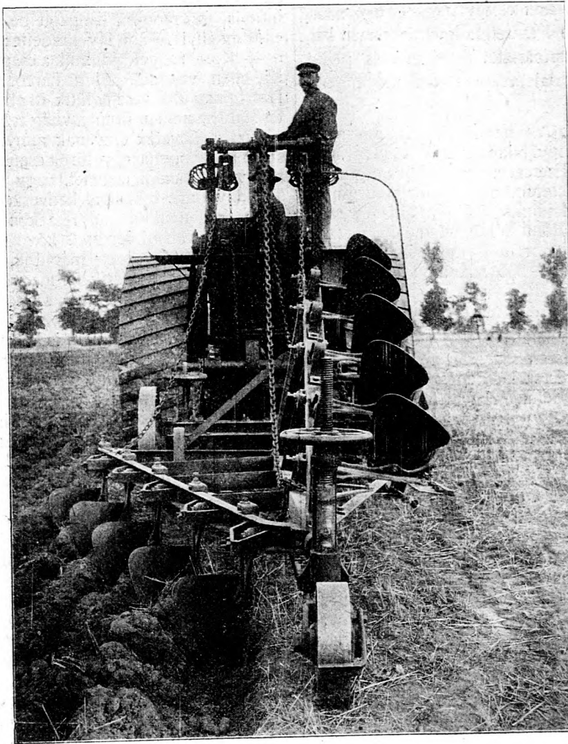
A Nicholson-féle gőz-szántógép hátulról.
