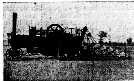
A Nicholson-féle gőz-szántógép oldalról.
