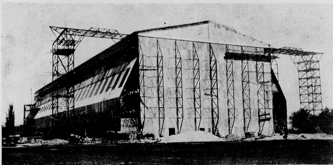
Zeppelin léghajója számára készült csarnok Metz városában. Innen megy Zeppelin legközelebbi útjára.
