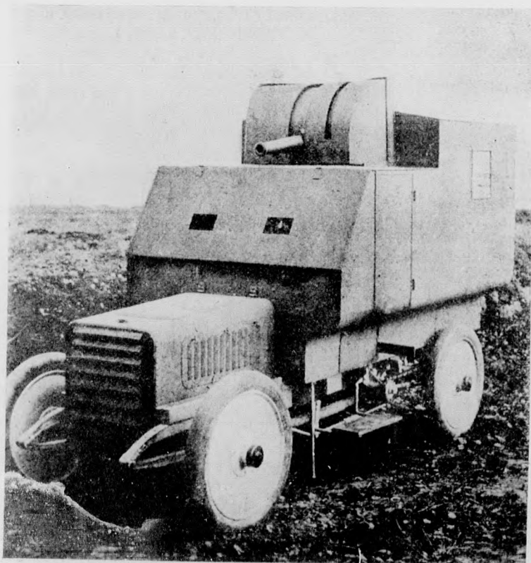
Érdekes haladás az ágyu ujtások terén. Képünk egy páncélos ágyu automobilt ábrázol, amely léggömbök ágyuzására készült.
