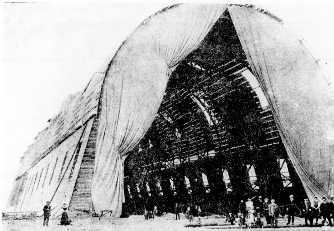
A «Deutschland» katasztrófája. A nagy léghajócsarnok Düsseldorfban, ahol a «Deutschland»-ot állandóan tartották.
