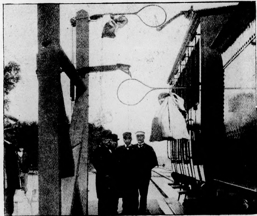
Postaszedő készülék.
