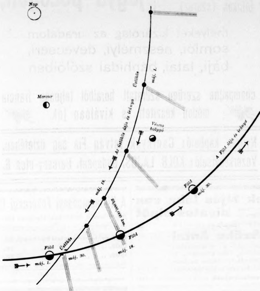
Képzünk az égi testek állását mutatja május hónapban. A vastagon húzott vonal a földnek, a vékonyabb a Halley-üstökösnek pályája. Az üstökös csóvjája mindenütt a naptól elfordított oldalon van. Máj. 18. a csóva éppen ráesik a földre.
