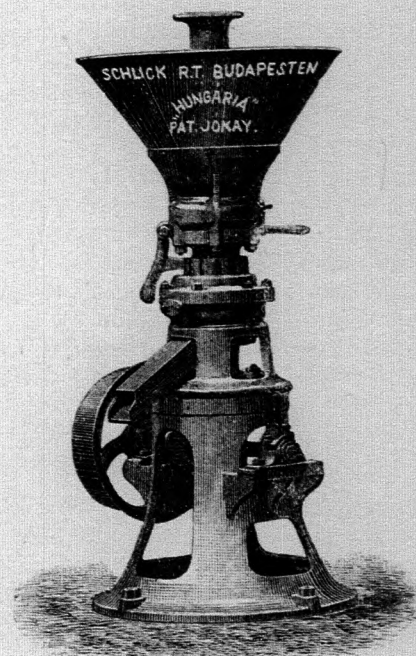
3. ábra. Hungária daráló gép.
