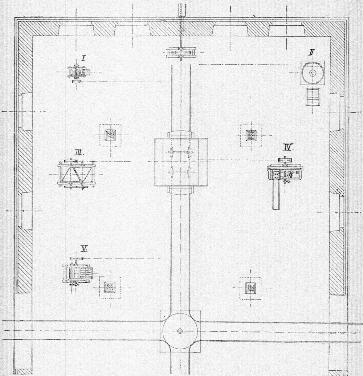
1. ábra. Takarmánykamra alaprajza.
