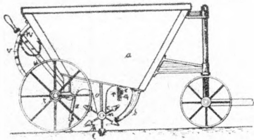
83. ábra. Burgonyaültető-gép oldalnézete
