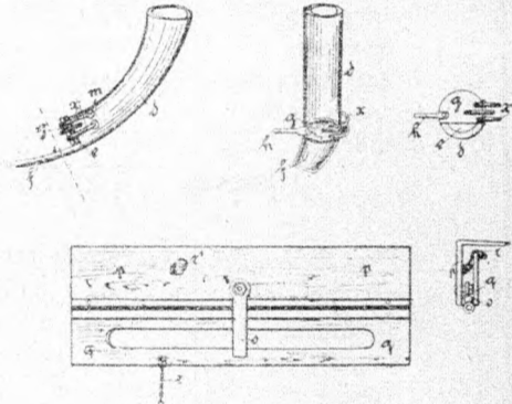
86. ábra. Burgonyaültető-gép egyes részletei.
