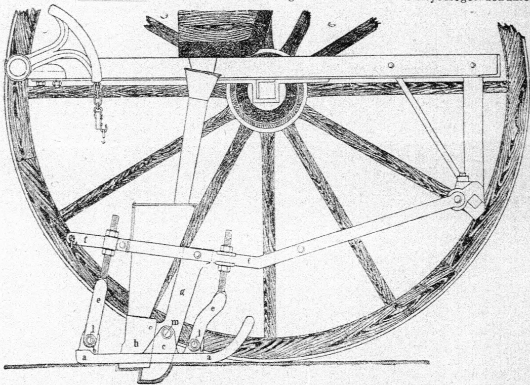
74. ábra. Negro-féle vetősaru-szán.
