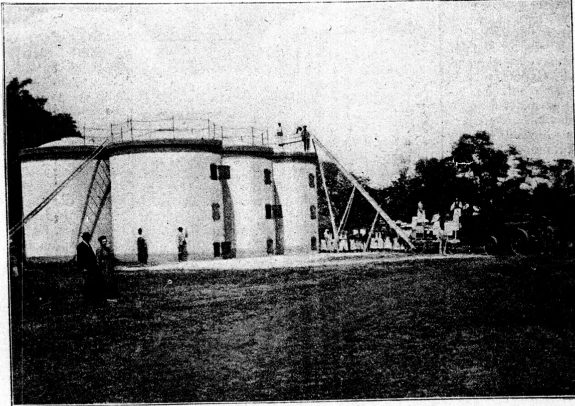
166. ábra. Téglából épült takarmánysziló a k.-nyéki uradalomban.
