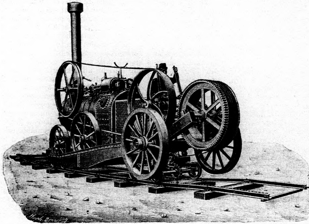
204. ábra. A gőzeke aparátus sodrony jobja.
