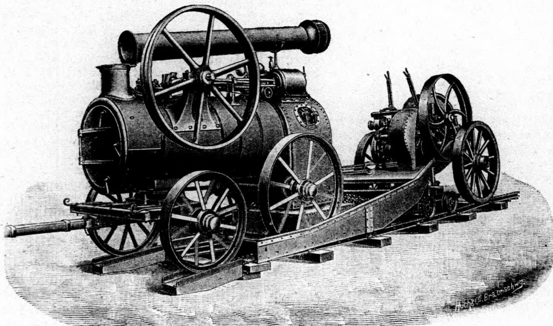
202. ábra. Lokomobilra alkalmazott gőzeke aparátus.
