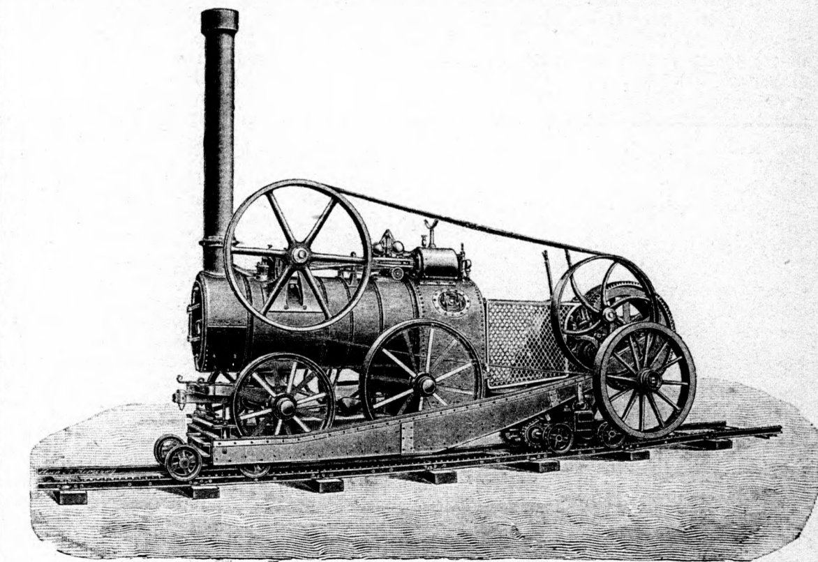
203. ábra. Lokomobil gőzszántásra felszerelve.
