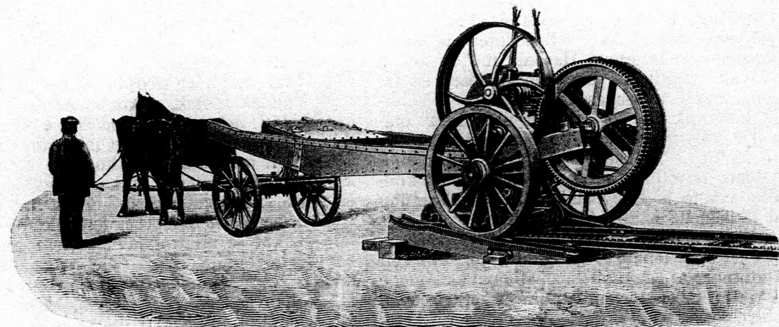
206. ábra. Lokomobil vaskocsija szállításra felszerelve.
