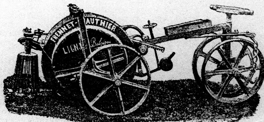
210. ábra. Frennet Wauthier-féle répakiemelőgép munkára beállítva.
