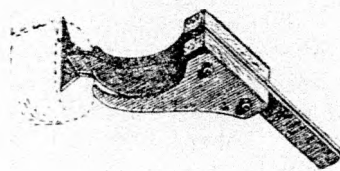
211. ábra. Frennet Wauthier-féle répakiemelőgép fejelszerkezete.
