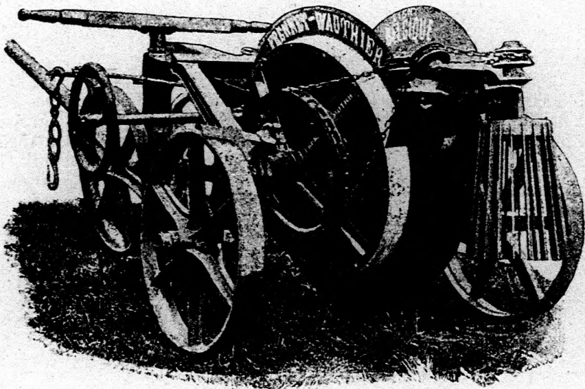
208. ábra. Frennet Wauthier-féle répakiemelőgép.
