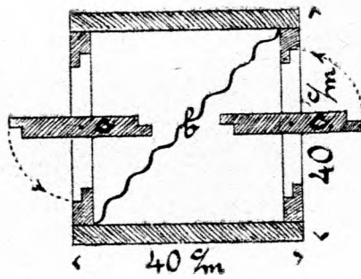
37. ábra. A szelelő alsó vége. b) bádoglemez, c, c, záróajtócskák.
