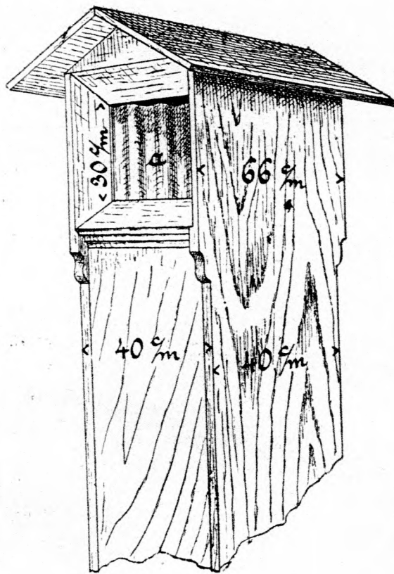
36. ábra. Istállószelelőtető készülék. a) A tölésészerű nyílás.
