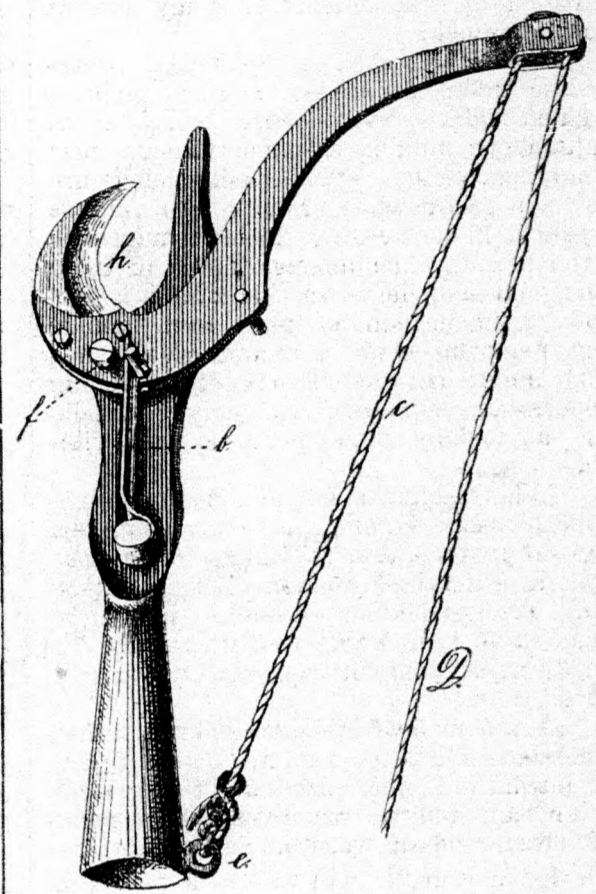
63. ábra. Felülről metsző hernyónyíró-olló.
