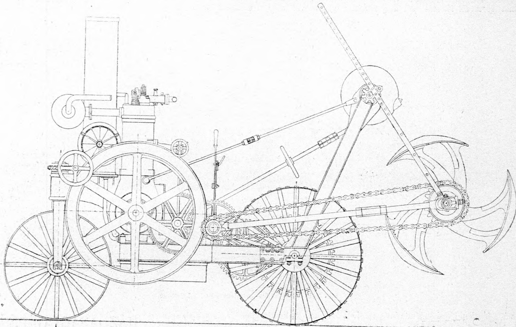
241. ábra. Mechwart-féle petroleum-eke oldalnézete.
