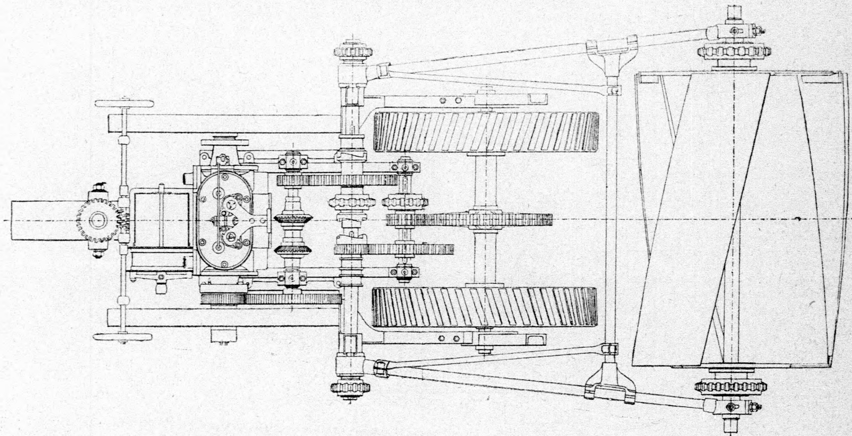
242. ábra. Mechwart-féle petroleum-eke felülnézetben.
