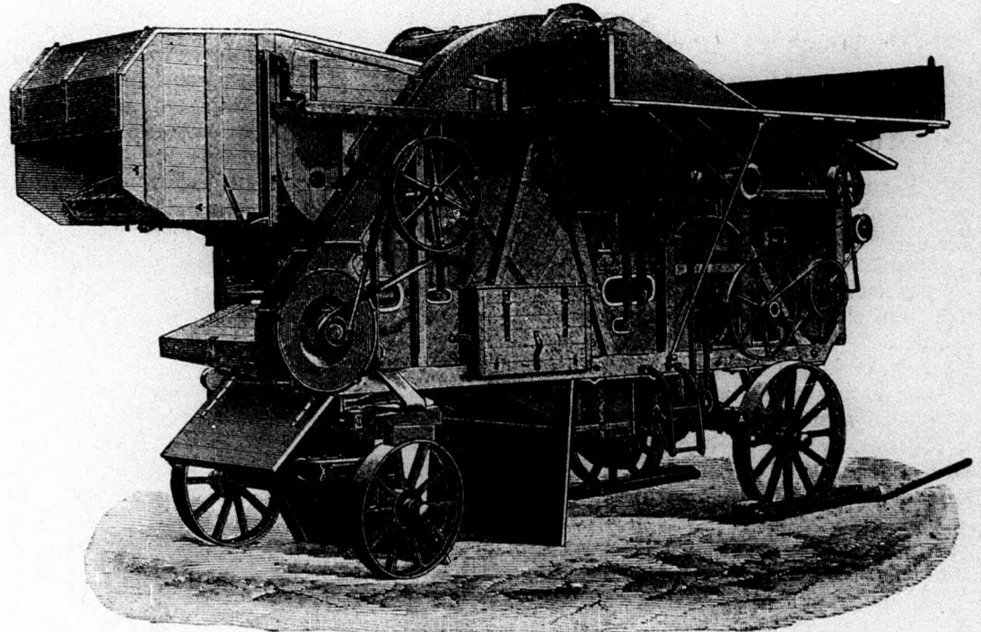
37. ábra. A Graepel-Marschall-féle kombinált löhere- és gabonacséplő-gép. Baloldali nézet.
