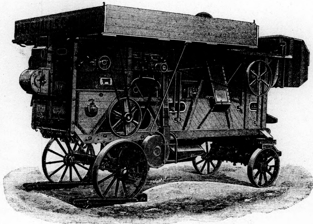
38. ábra. A Graepel-Marschall-féle kombinált löhere és gabonacséplő-gép. Jobboldali nézet.
