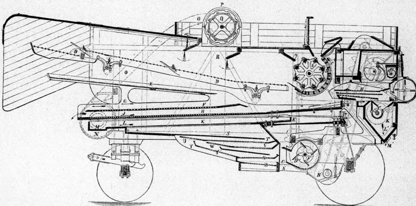
36. ábra. A Graepel-Marschall-féle szab. kombinált lóhere és gabonacséplőgép. Hosszmetszet.
