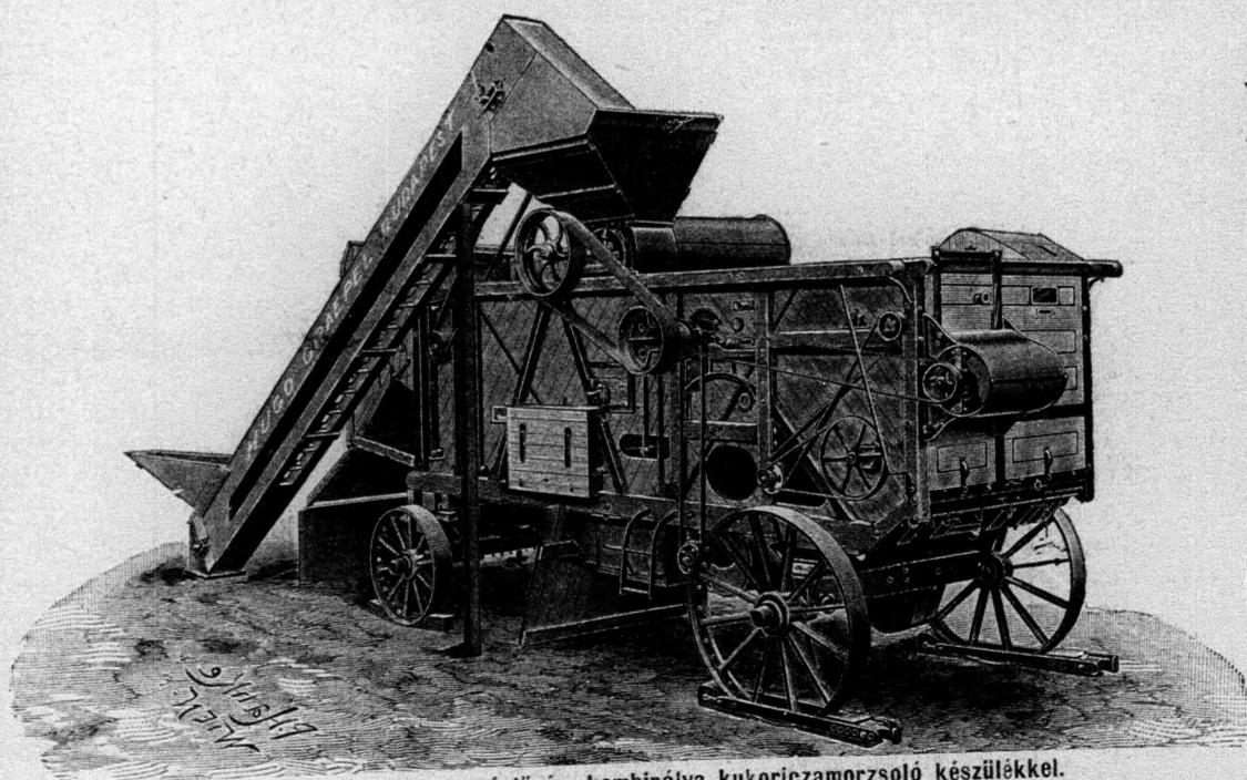
MARSHALL-féle gabona cséplőgép, kombinálva kukoriczamorzsoló készülékkel.
