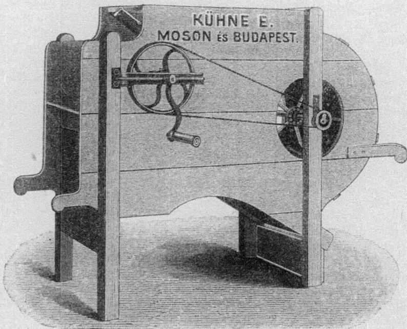
114. ábra. Kühne E. I. sz. szelelője.
