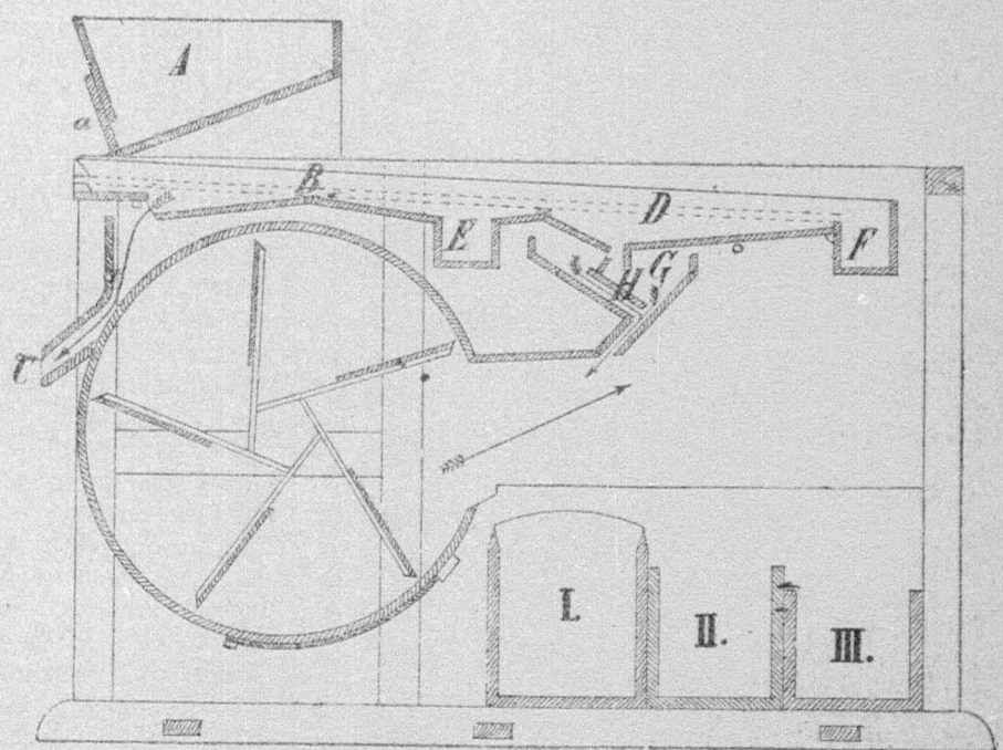
118. ábra. A Behán S.-féle terményrosta. Hosszmetszet.
