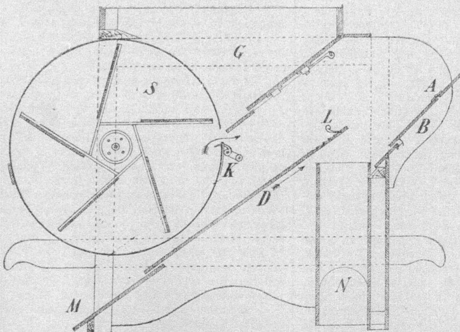
117. ábra. Kalmár Zs. „Ideal C” nevű szelelője. Hosszmetszet.
