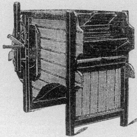
116. ábra. Kalmár Zs. „Ideal C” nevű szelelője.
