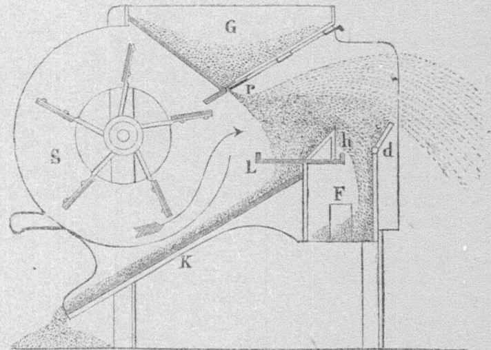
115. ábra. Kühne E. I. sz. szelelője. Hosszmetszet.
