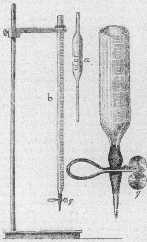
122. ábra. Sav-meghatározó.
