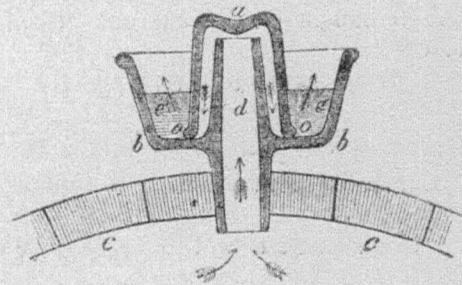
123. ábra. Erjesztő-tölcsér.
