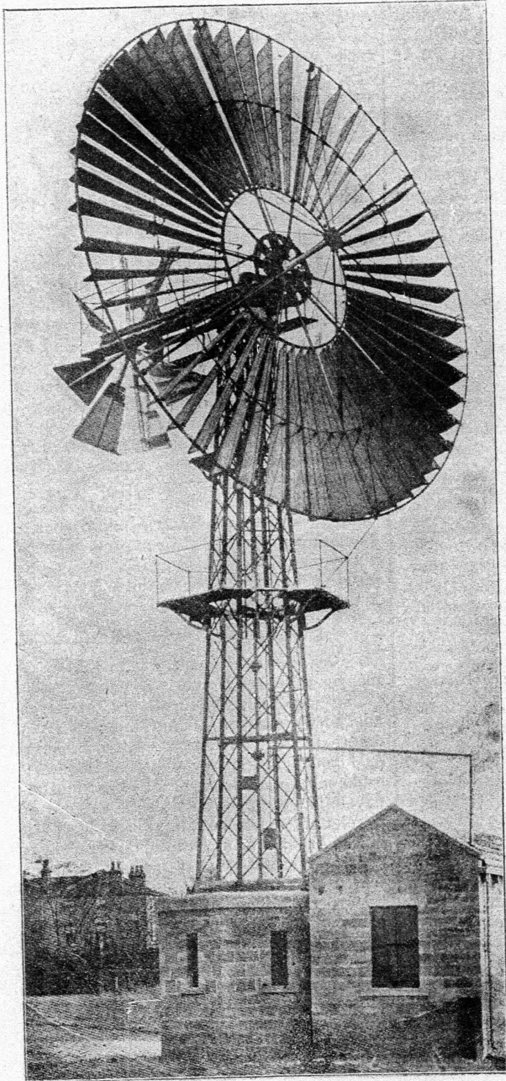
60. ábra. Szélmotor villamvitágítási célra Boyle-Hall-ban.
