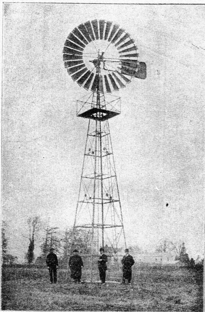
61. ábra. „Hercules” szélmotor Hardingsstone mellett.
