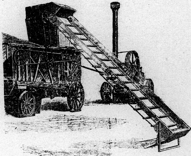
40. ábra. Golwer-féle távetető földre állítva.
