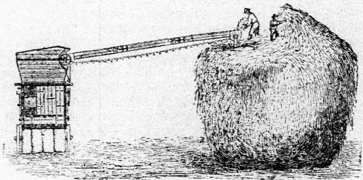
39. ábra. Golwer-féle távetető asztalmagasságra állítva.
