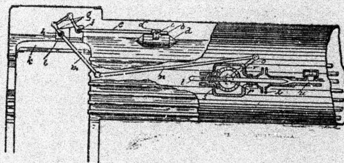
245. ábra. Önműködő vízszabályozó hosszmetzetben.
