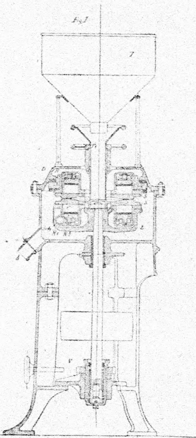
15. ábra. Az „Ottynia“ daráló és őrlő malom szerkezeti elrendezése.
