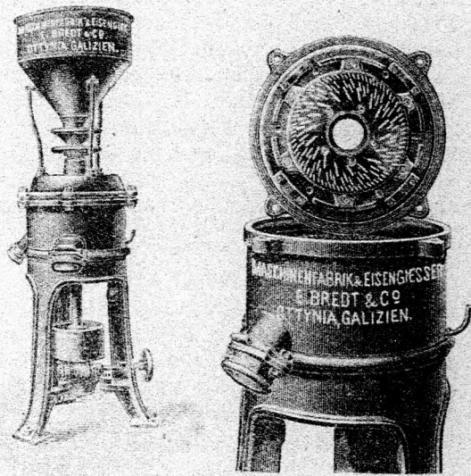
16. ábra. Az „Ottynia“ daráló és őrlő malom nézete és őrő szerkezete.
