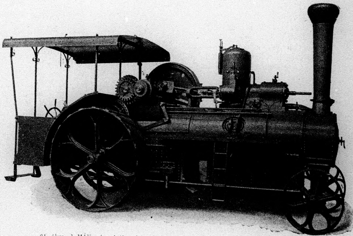
61. ábra. A MÁV. gépgyárában készült MB. jegyű kéthengeres „Compound” közuti mozdony.
