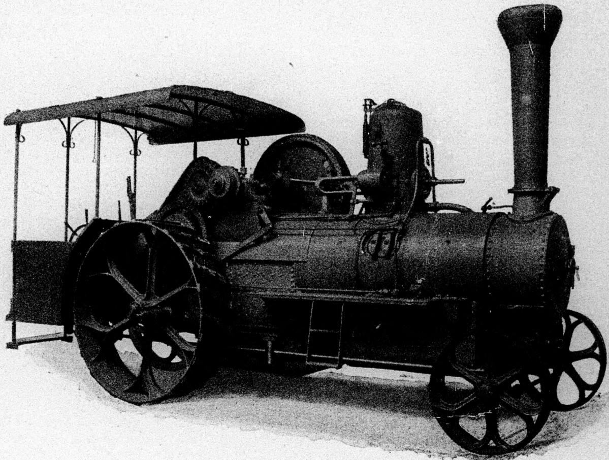
62. ábra. A MÁV. gépgyárában készült MBB. jegyű egyhengeres közuti mozdony.
