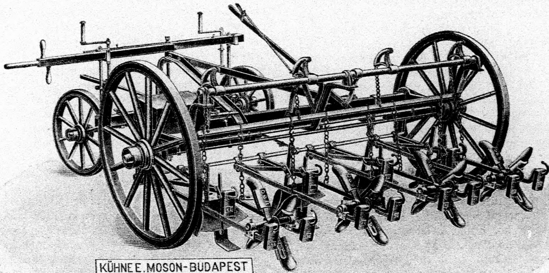
126. ábra Kühne E. burgonyalyukgató (fészekvályó) gépe.
