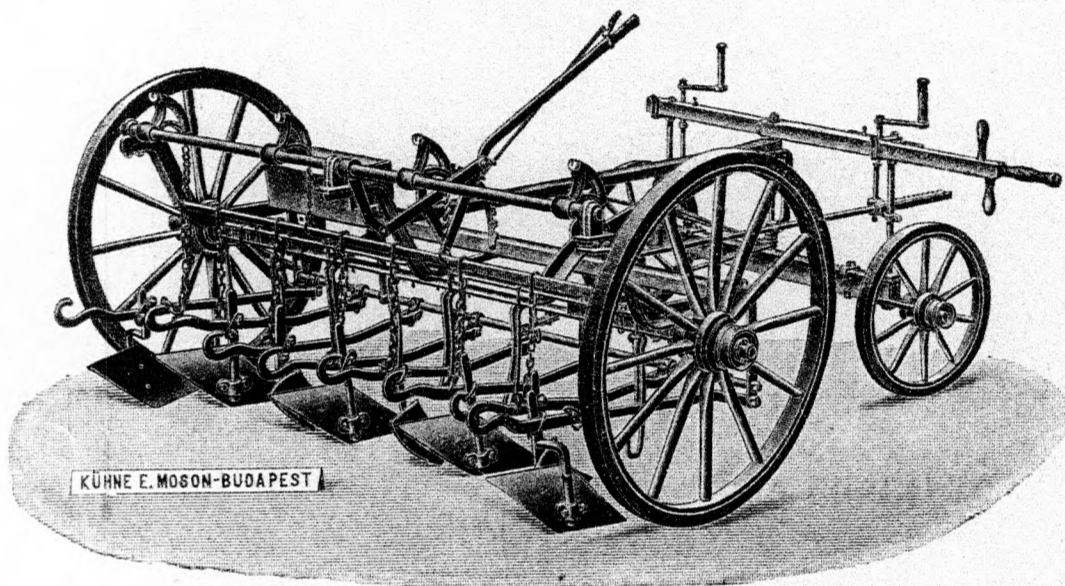
128. ábra. Kuhné E. burgonyatakaró gépe.
