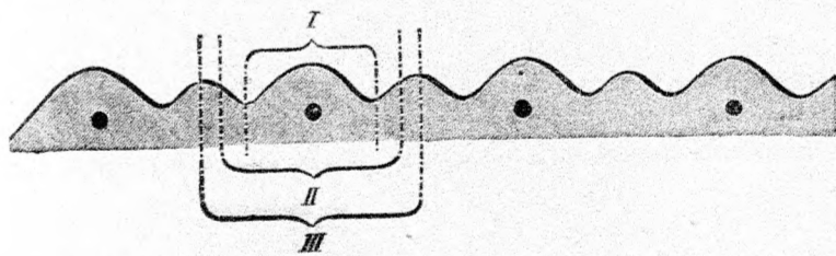
129. ábra. A talaj felszine a Kuhné E. burgonyatakaró gépe után.
