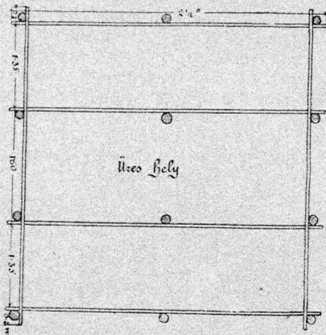
157. ábra. Ideiglenes kettős göré alaprajza.
