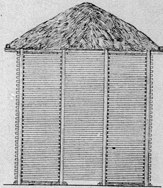
158. ábra. Ideiglenes kettős göré.
