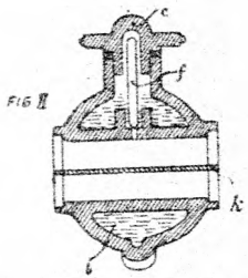
42. ábra. Olajkamrás csapágyak nézetben és hossz-metszetben.
