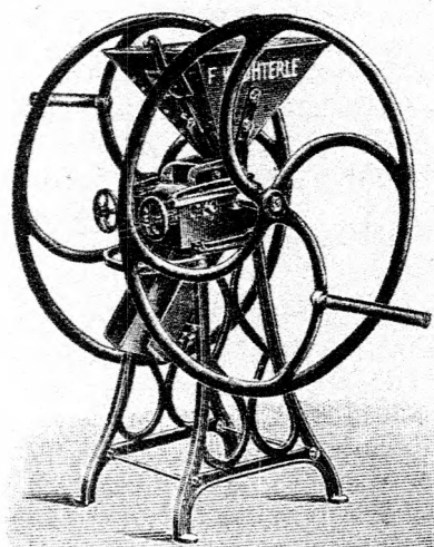
44. ábra. Kézi daráló rázómuvel.
