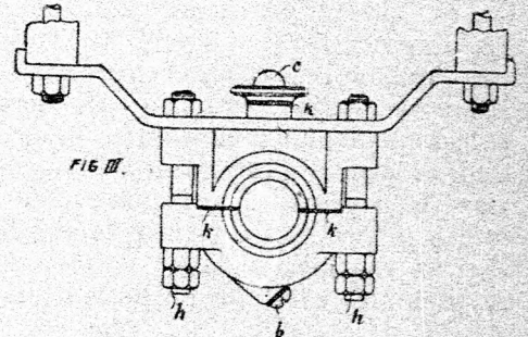
40. ábra. Olajkamrás csapágyak méretben és hossz-metszetben.
