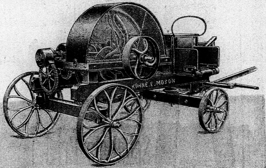
„M. 66.“ Jegyű szecskavágó szállítóeszközzel, munkabrása 1200—2000 kg. óránként, ára 860 korona.
