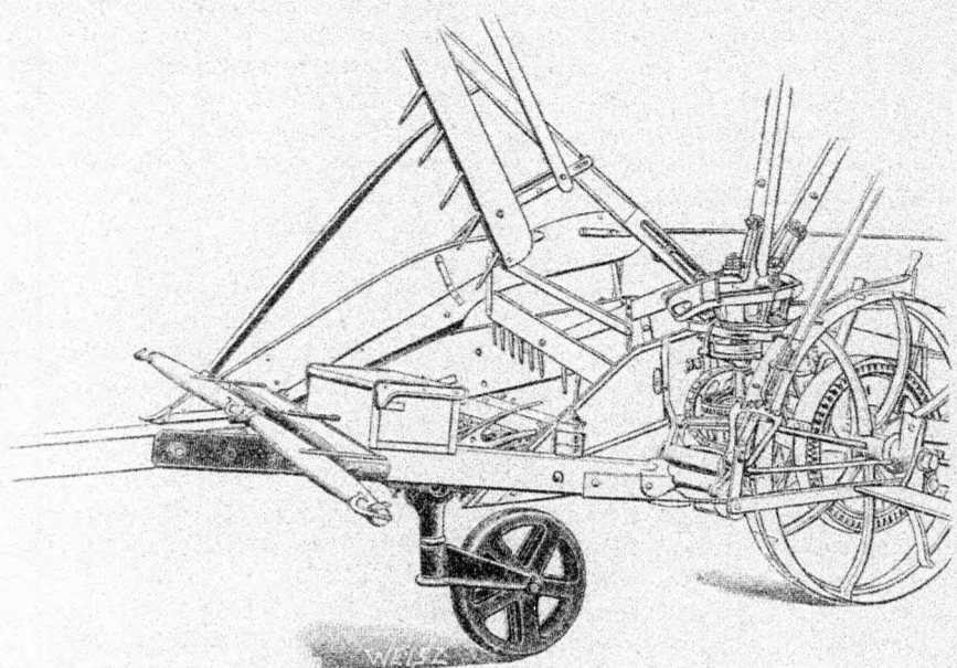
105. ábra. Mankóskerektű rudhordó.
