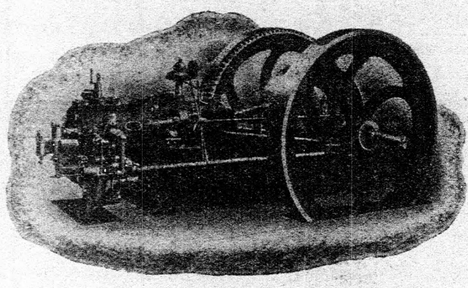
Egy 6-5 HP. NYERSOLAJMOTOR és egy 21 HP. BENZINLOKOMOBIL a TECHNOLOGIAI IPARMUZEUMBAN (Budapest, VIII., József-körút 6. szám.) ÜZEMBEN megtekinthető.
