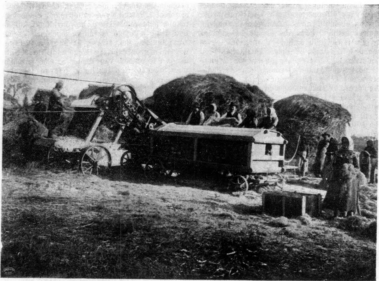
16. ábra. Kettős rendszerű olasz kenderkimunkáló gép a lokomobil felől nézve. Balról a törő gép, jobbról a tiloló szerelvény.
