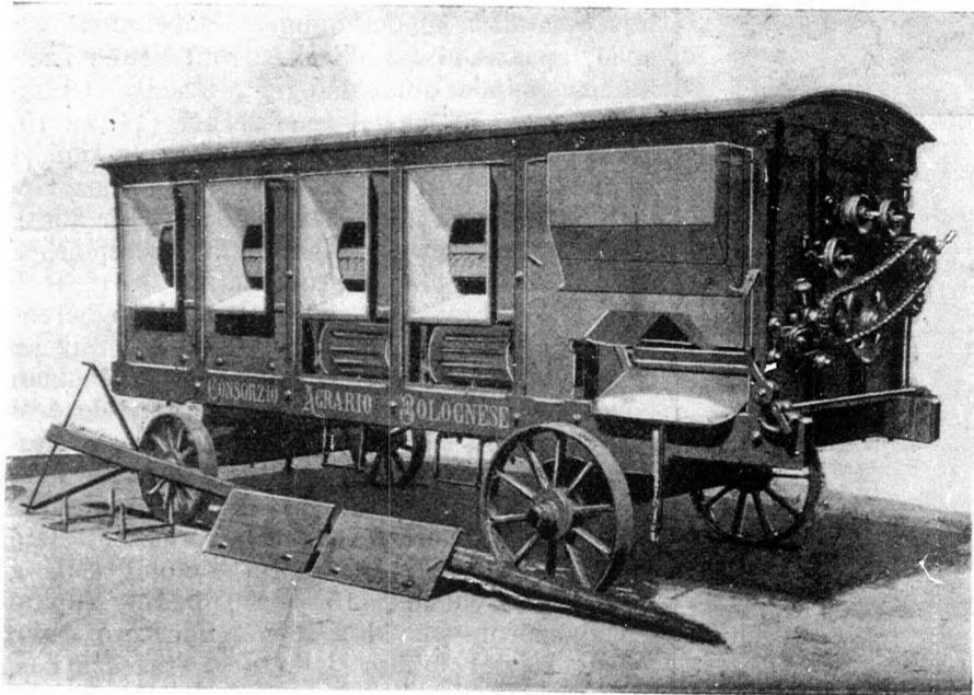
14. ábra. Egyes rendszerű olasz kenderkimunkáló-gép. Jobbról alul a törő részesz etető nyílása.
