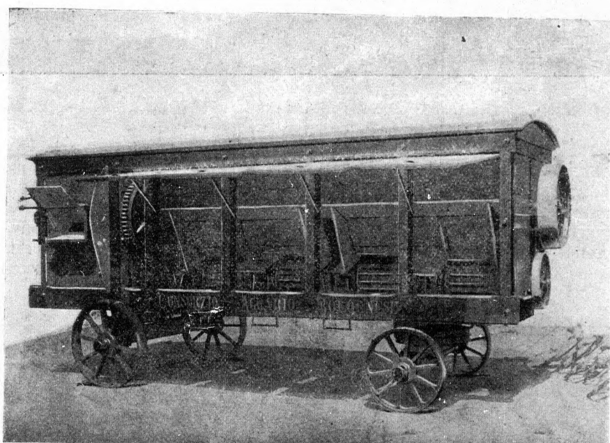
5. ábra. Egyes rendszerű olasz kenderkimunkáló-gép. Balról az etető rekesz ki-szájadzása, jobbról négy tiloló rekesz etető nyílása.
