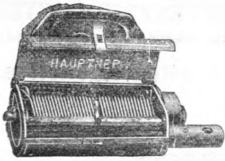
13. ábra. Hauptner H. állattisztító-gépe nyitva.
