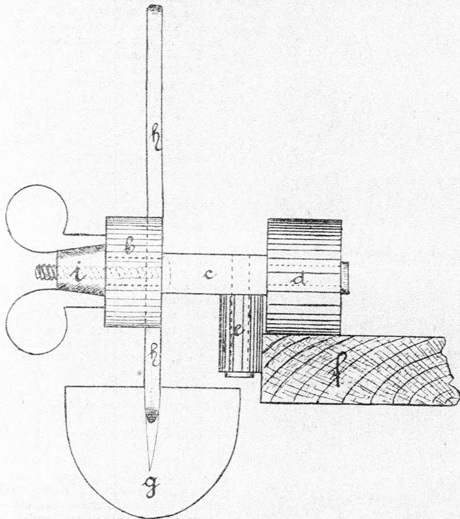
37. ábra. Legány-féle magárokkihuzó kapa előnézete. Természetes nagyságban.
