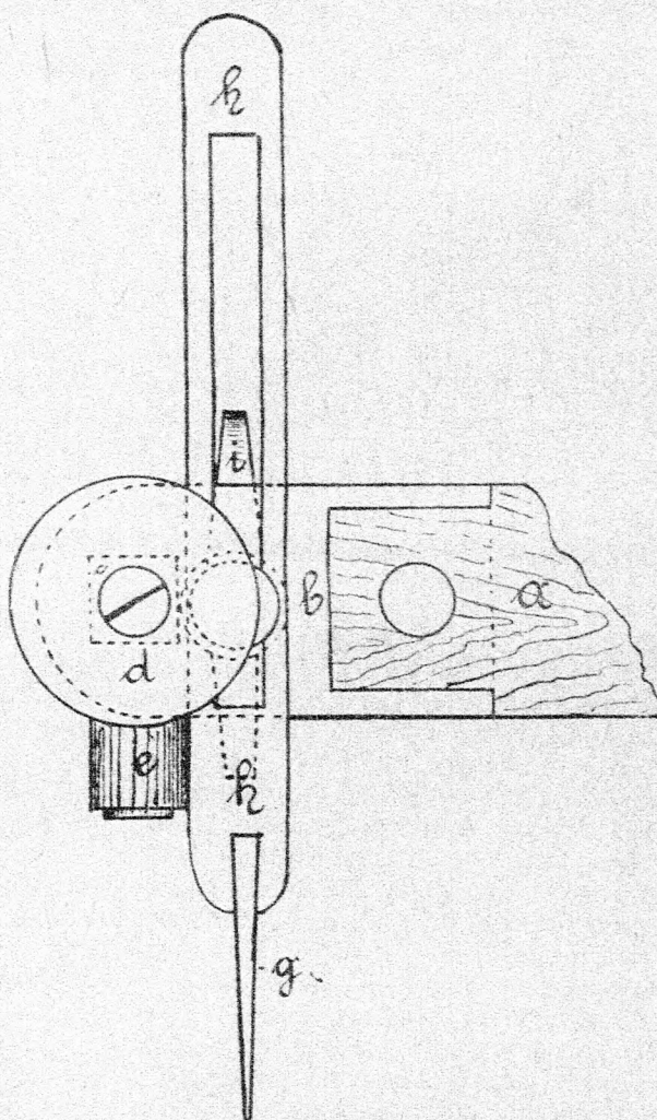
38. ábra. Legány-féle magárokkihuzó kapa oldalnézete. Természetes nagyságban.
