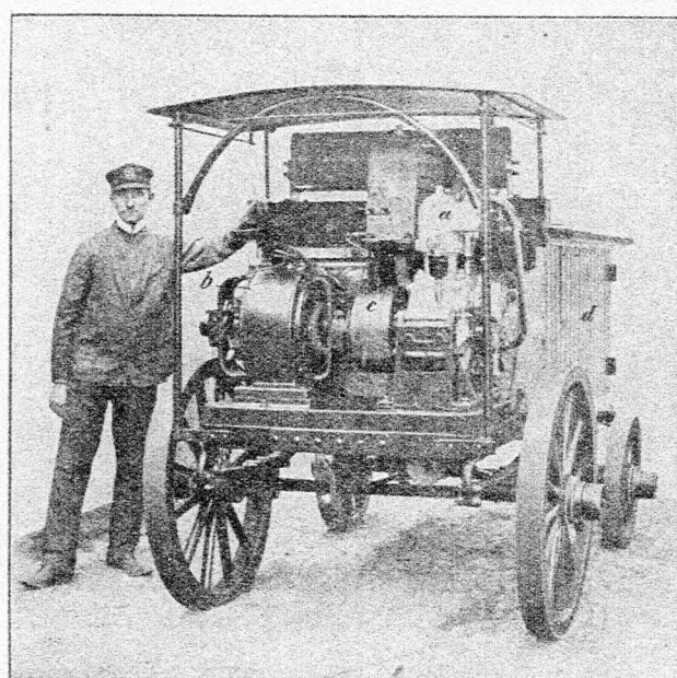
16 20 lóerejű elektro-lokomobil.
