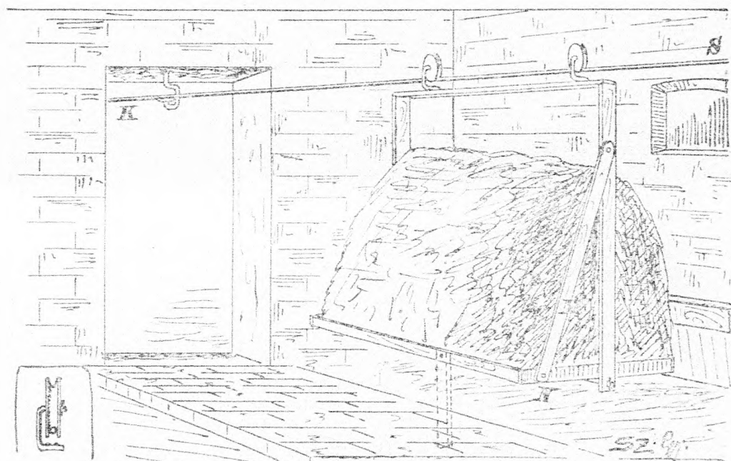
56. ábra. A függő trágyakocsi szerkezete.
