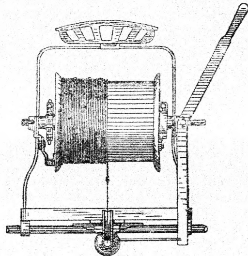
64. ábra. Sodronyvezeték a „Senior“ tengerültető gépen.
