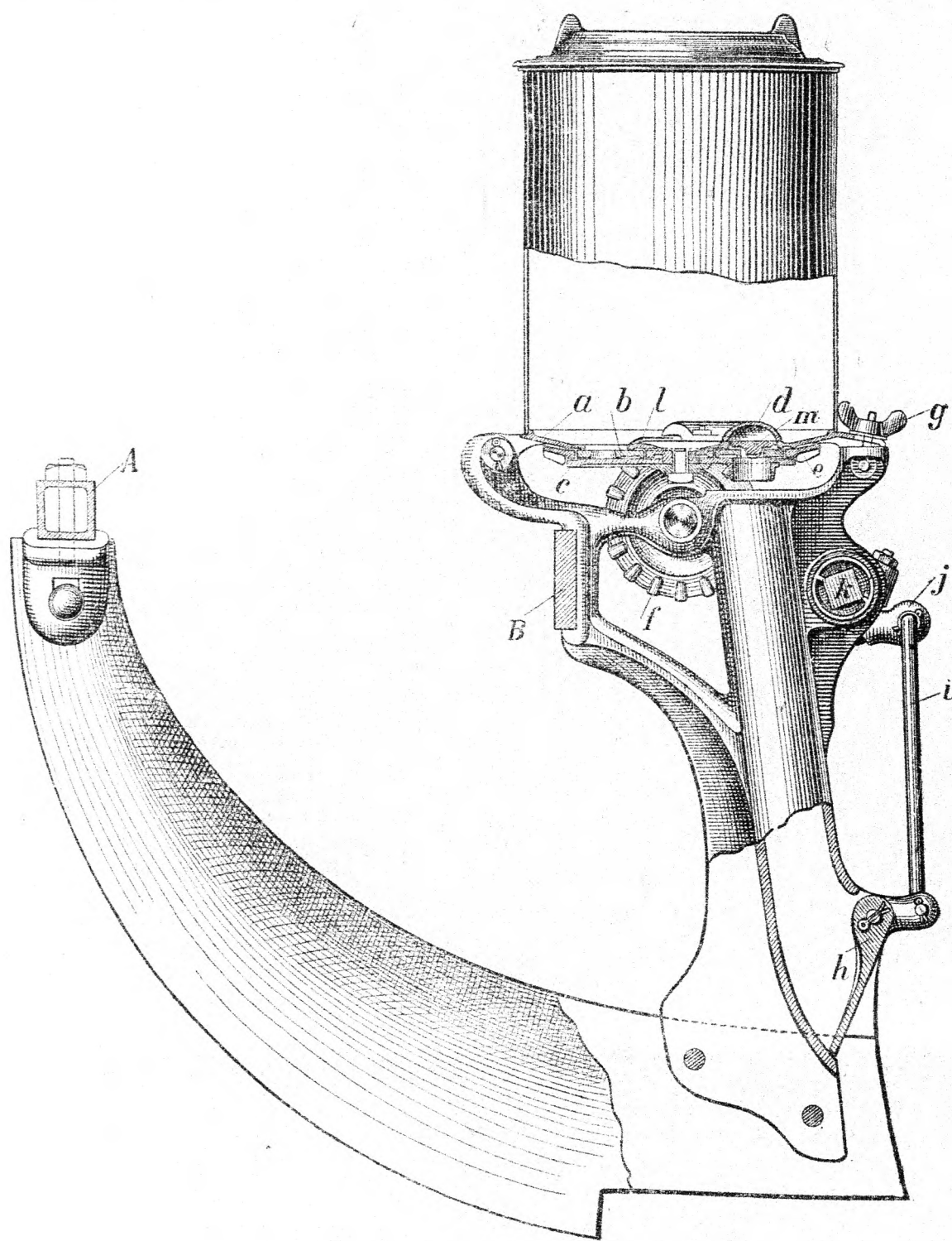
61. ábra. A „Senior“ tengerültető gép vetőkészüléke.
