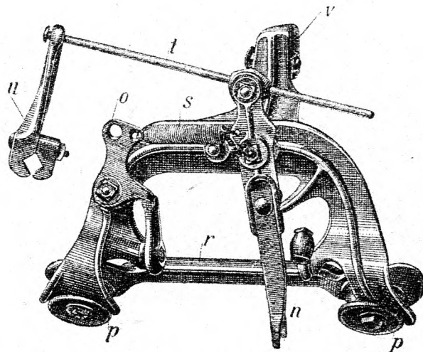
60. ábra. A „Senior“ tengerivetőgép vetőszelep-nyitója.
