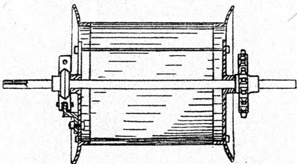
63. ábra. Sodronydob a „Senior“ tengerültető gépen.
