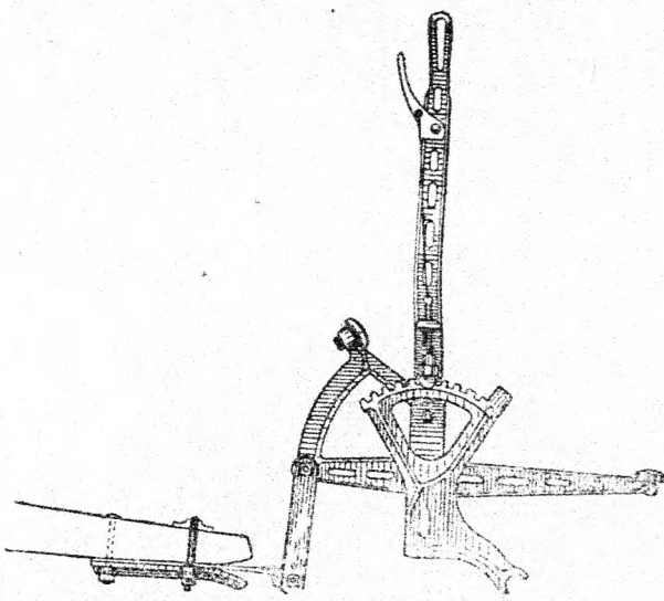
62. ábra. Kiemelő a „Senior“ tengerültető gépen.
