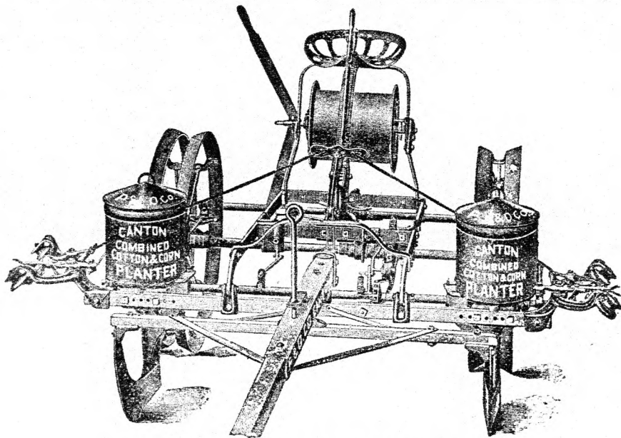
„Senior“ tengeri-ültetőgép autom. négyzet-ültetőkészülékkel.
