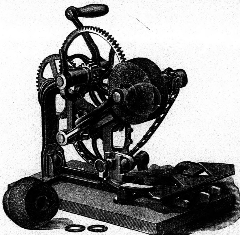
„Western“ aratógépkés köszörülésre beállítva.
