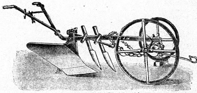
78. ábra Jurenák-féle IV. számú eke.
