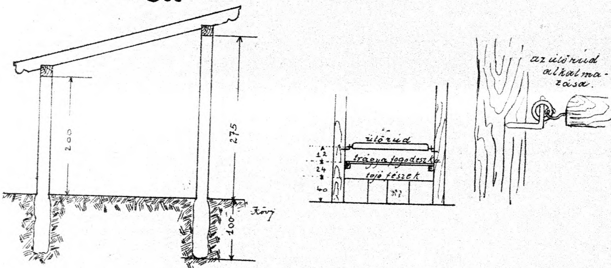
74. ábra. Baromfiólrészek oldalnézete.
