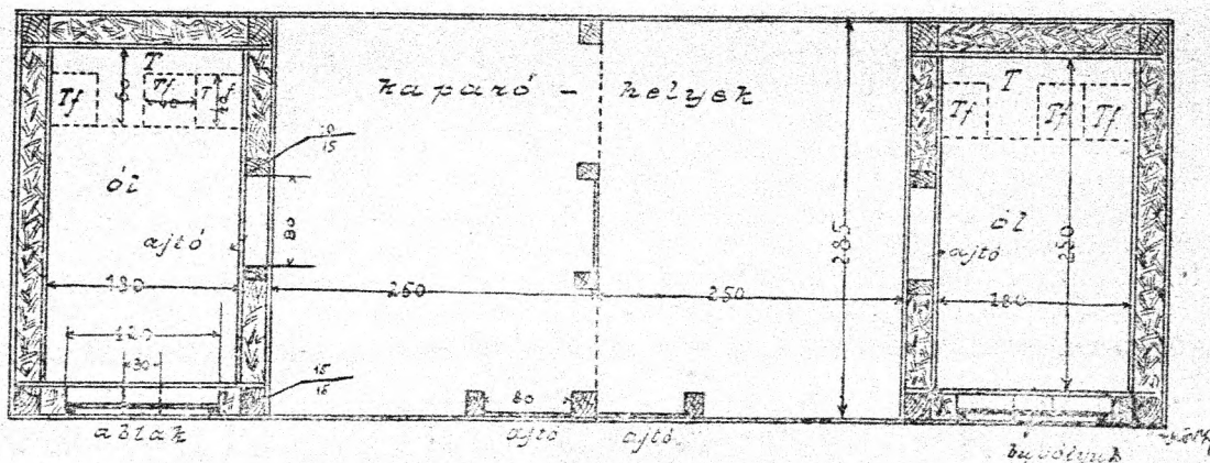
76. ábra. Baromfi-helyiség alaprajza.
