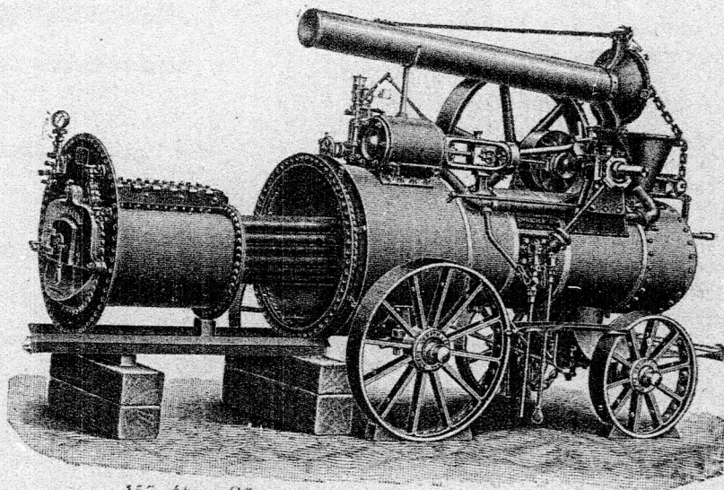
157. ábra. Gőzmozgony kihuzható csöveskazánál.
