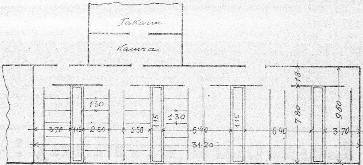
160. ábra. Keresztállású ököristálló 48 darabra.
