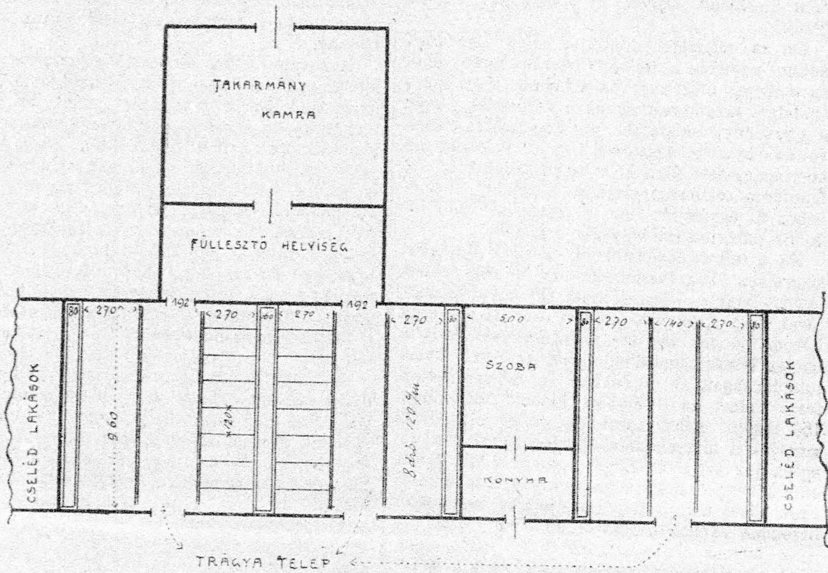
158. ábra. Régi istálló berendezés.
