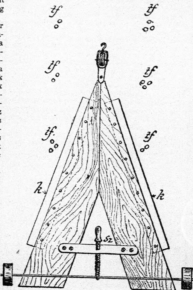
198. ábra. Teleki Arvéd gróf tengeriszárlevágó-készüléke. k, k = kések; tf. = tengerifészek; sz = levágási magasság szabályozója.
