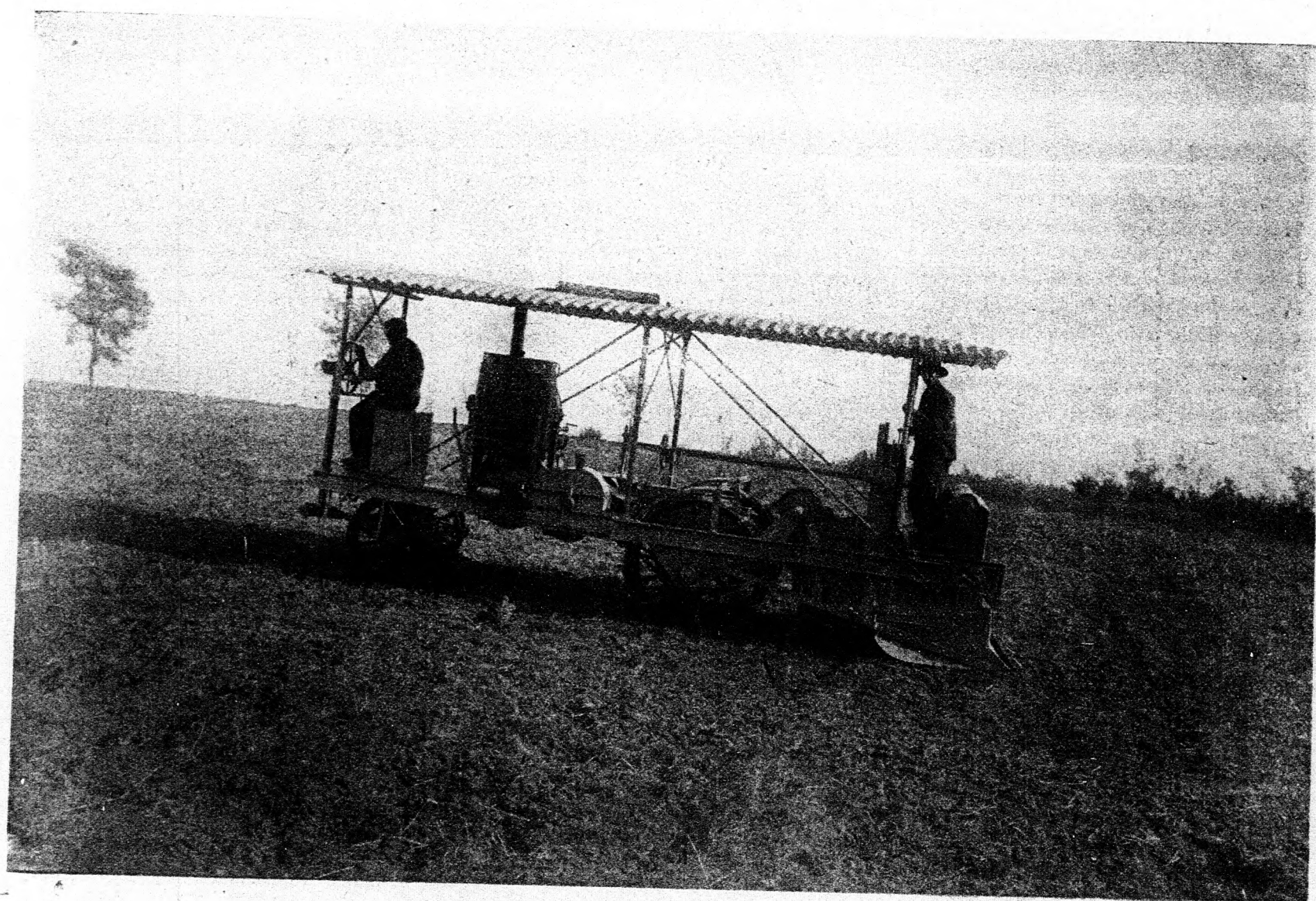
227. ábra. A Kőszegi-féle motoros talajmivelő gép munkára készen.
