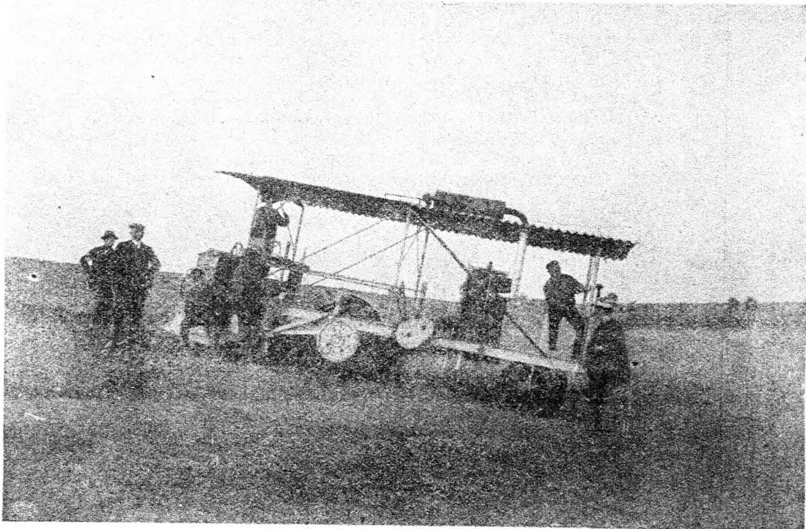
222. ábra. A Kőszegi-féle motoros talajművelő gép lejtőn lefelé állva. A gép elején látható a háromhengeres benzinmotor.
