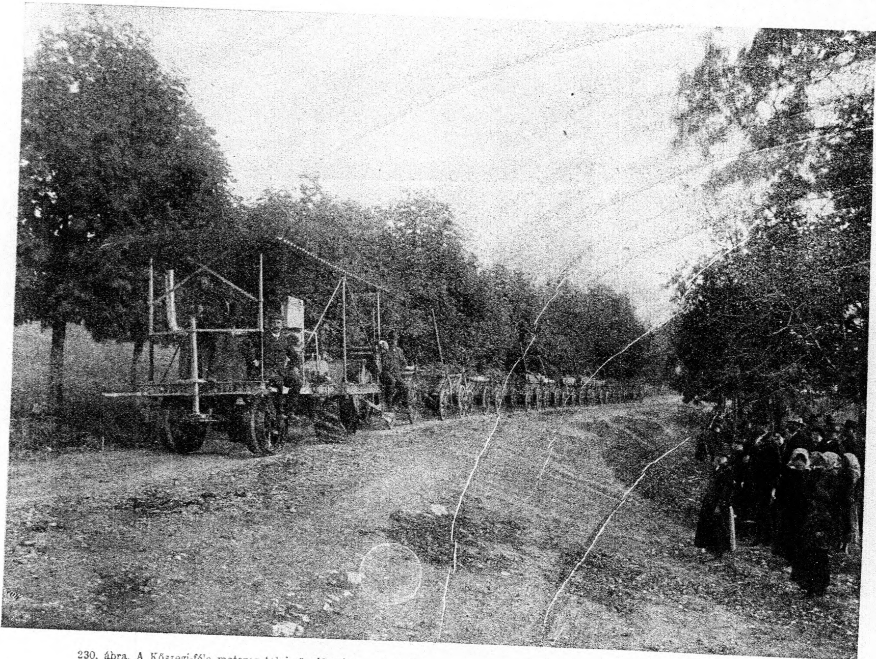
230. ábra. A Kőszegi-féle motoros talajművelő mint vontatógép, 3196 métermáza terhet (tizenkét megrakott szekeret) vontatva.
