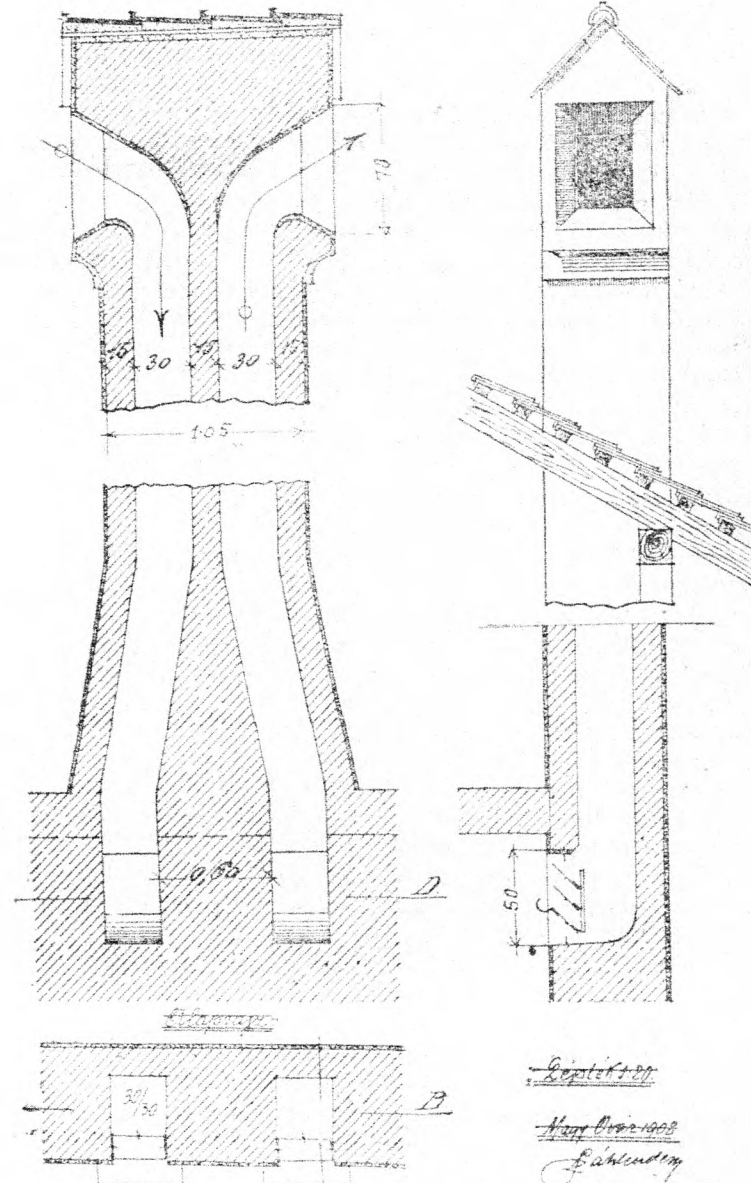
252. ábra. Kettős működésű istálló-szellőző kürtő téglaiból falazva.
