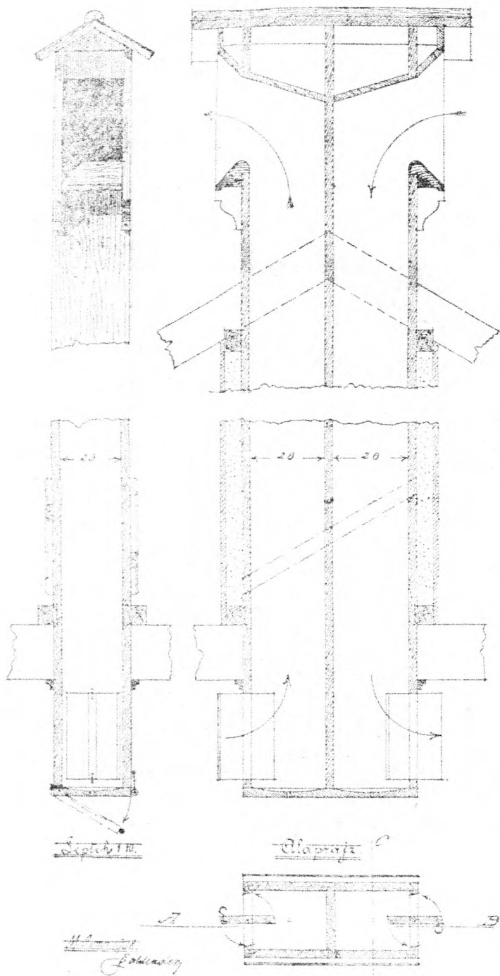
251. ábra. Kettős működésű istálló-szellőző kürtő deszkából készítve.
