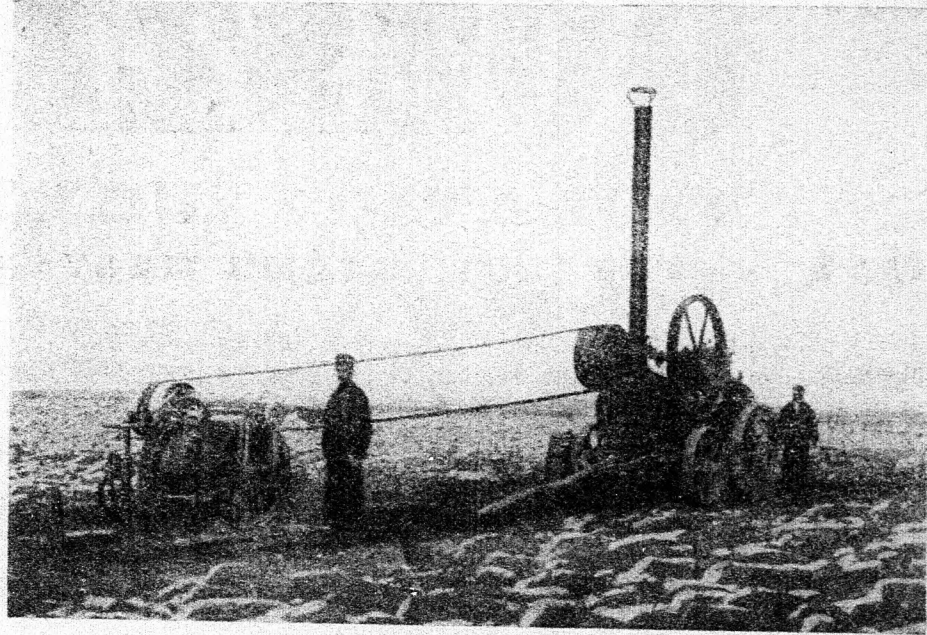
7. ábra. Kötélkapcsoló beiktatva.
