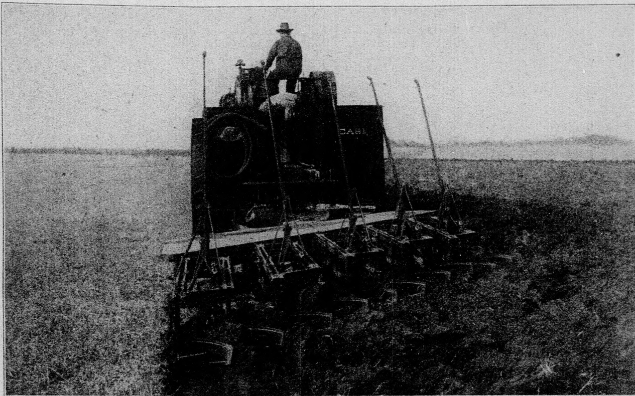
163. ábra. „Case“ amerikai gőzeke.
