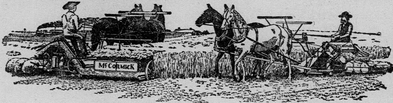
Mc Cormick kévekötaratógép 5 és 6 angol láb metszőszélességgel.
