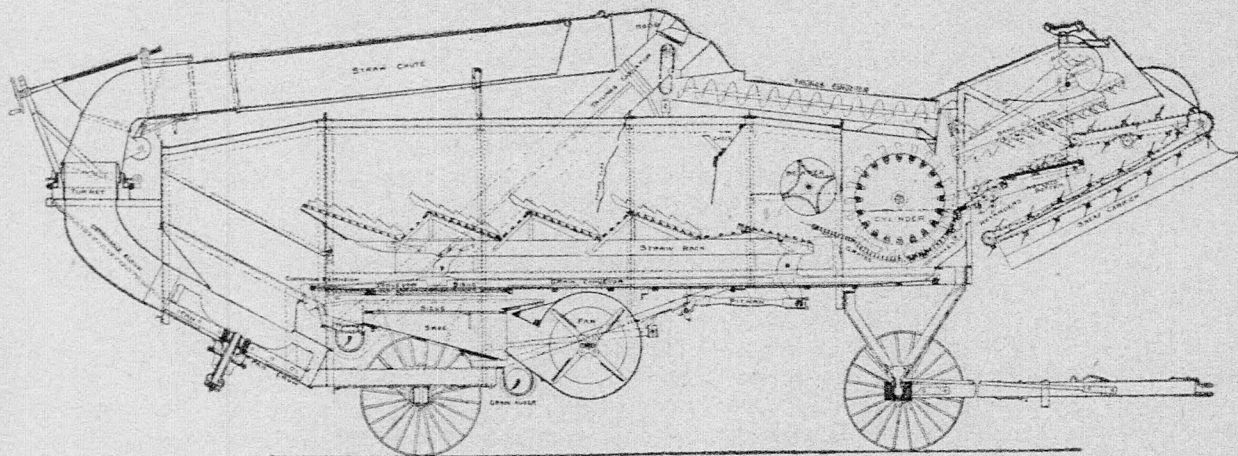
160. ábra. „Case” automatikus cséplőgép hosszmetsete.
