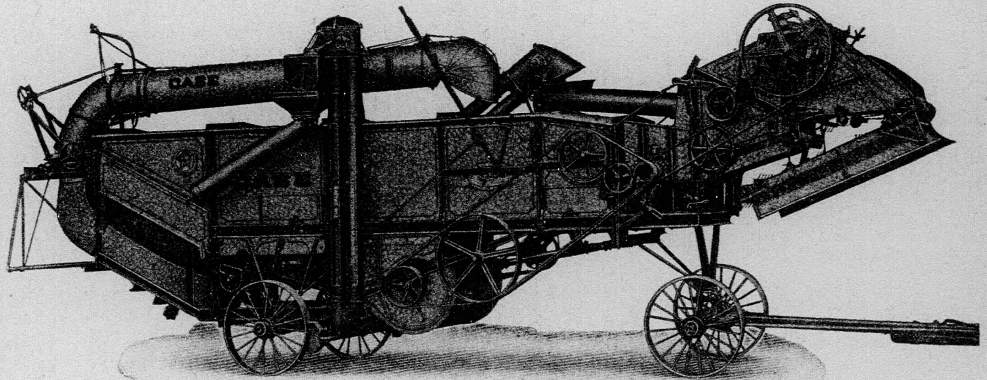
161. ábra. „Case” automatikus aczélszéplőgép önműködő gabonamérleggel.
