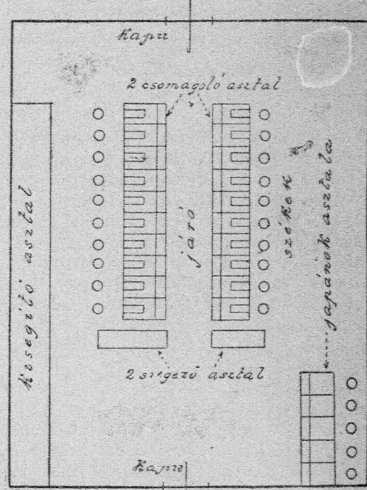
115. ábra. Gyümölcscsomagoló szin keresztmetszete és alaprajza.
