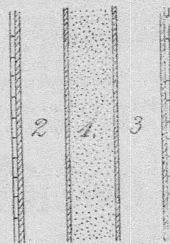
111. ábra. Gyümölcsraktár fal elszigetelése.
