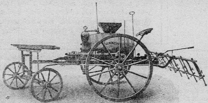
Állítható 9-soros répapermetező.
