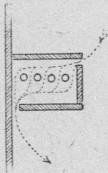
114. ábra. Hűtőcsövek a raktárfal mentén.
