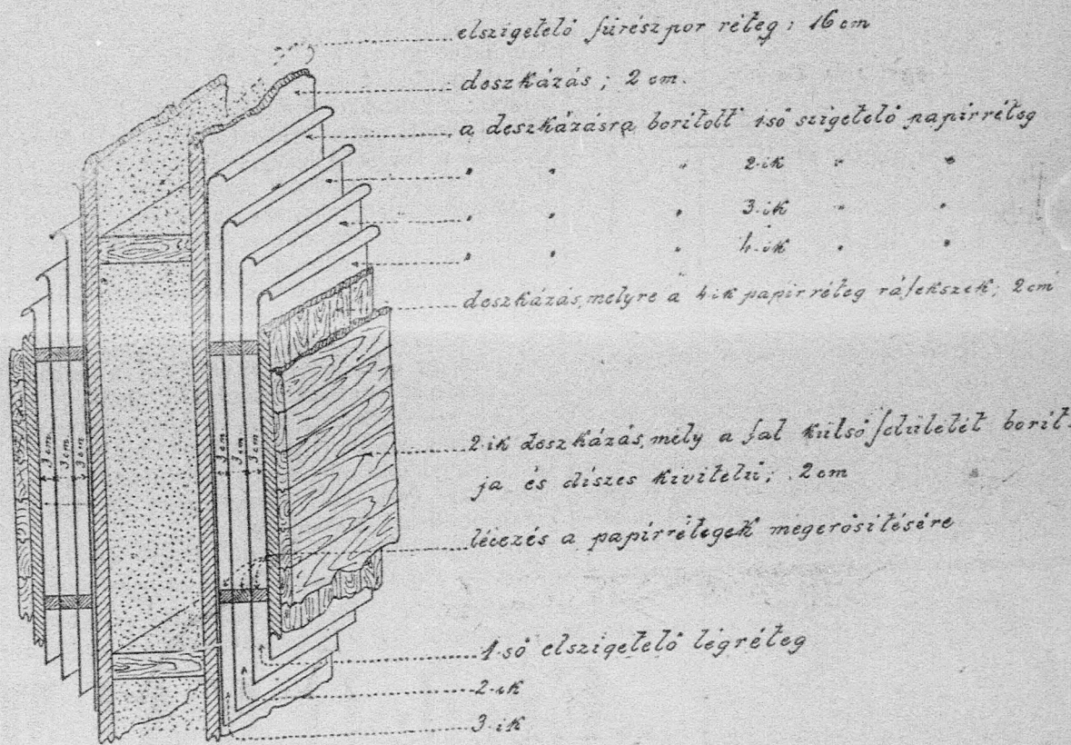
A fal másik oldala ugyanilyen elrendezéssel bír. 112. ábra. Gyümölcsraktár falának átnézete.
