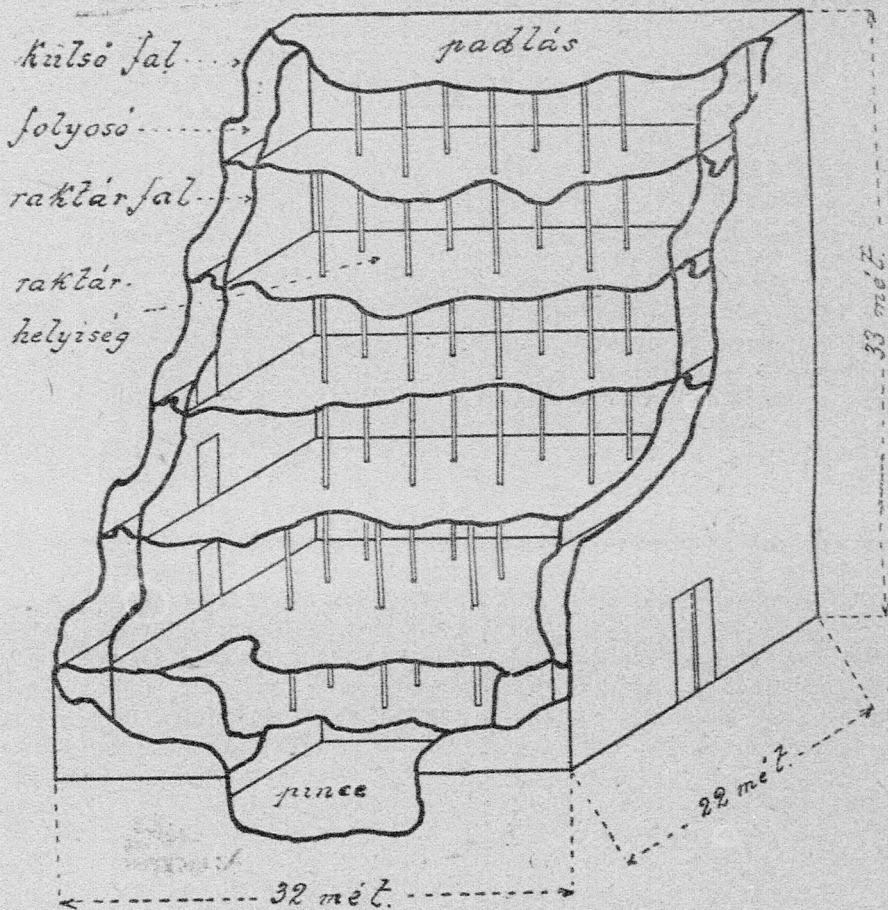
110. ábra. Gyümölcsraktárépület átnézete.
