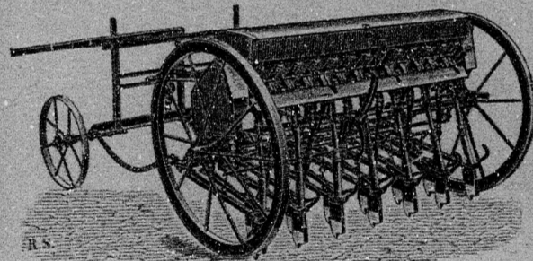
Valódi „SACK”-féle sorbavetőgép.
