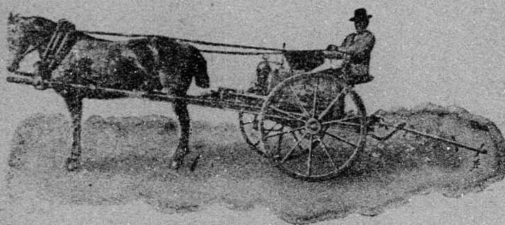
Vadrepcze- és burgonyapermetező, 5 méter munkaszélességgel
