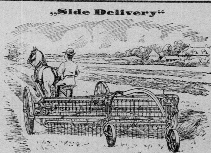
„Side Delivery“ Kombinált szénagyűjtő- és forgatógép.
