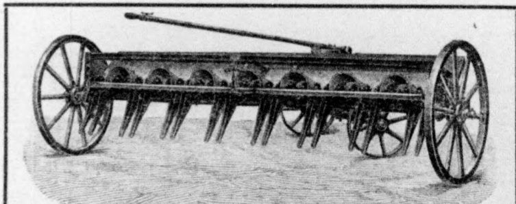
Szabad. autom. chilisalétromszóró, melylyel chili, őrlés nélkül szórható. Kapható: 2-sorosan taligaalakban, egy igavonó részére 3-8-sorosig.
