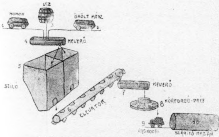
170. Ábra. Mészhomok-tégla gyártási folyamata.
