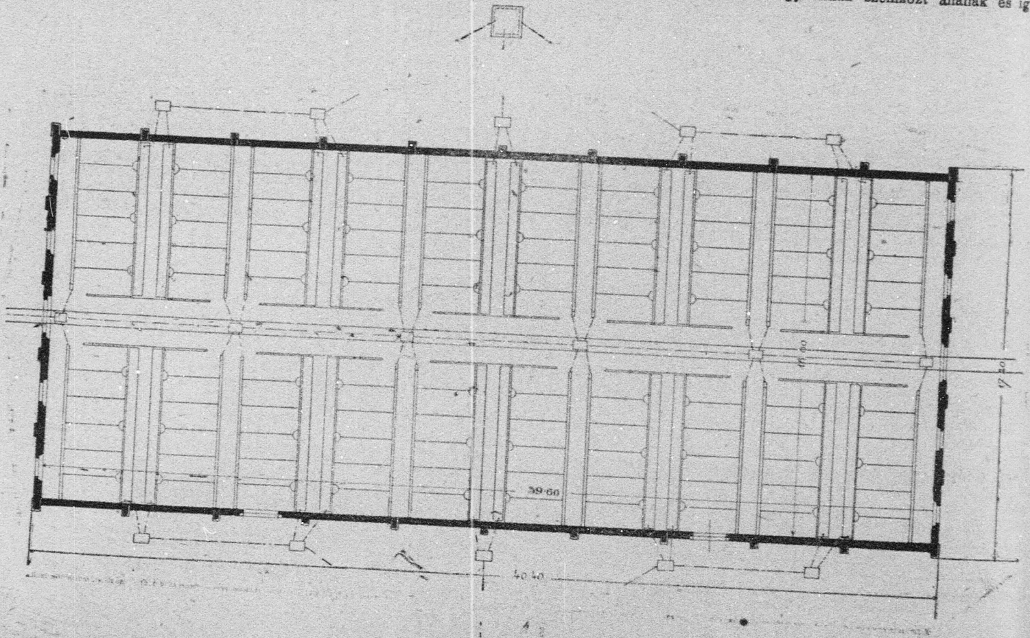
73. ábra. Modern berendezésű vasbetonistálló 120 tehénre. (Alaprajz.)
