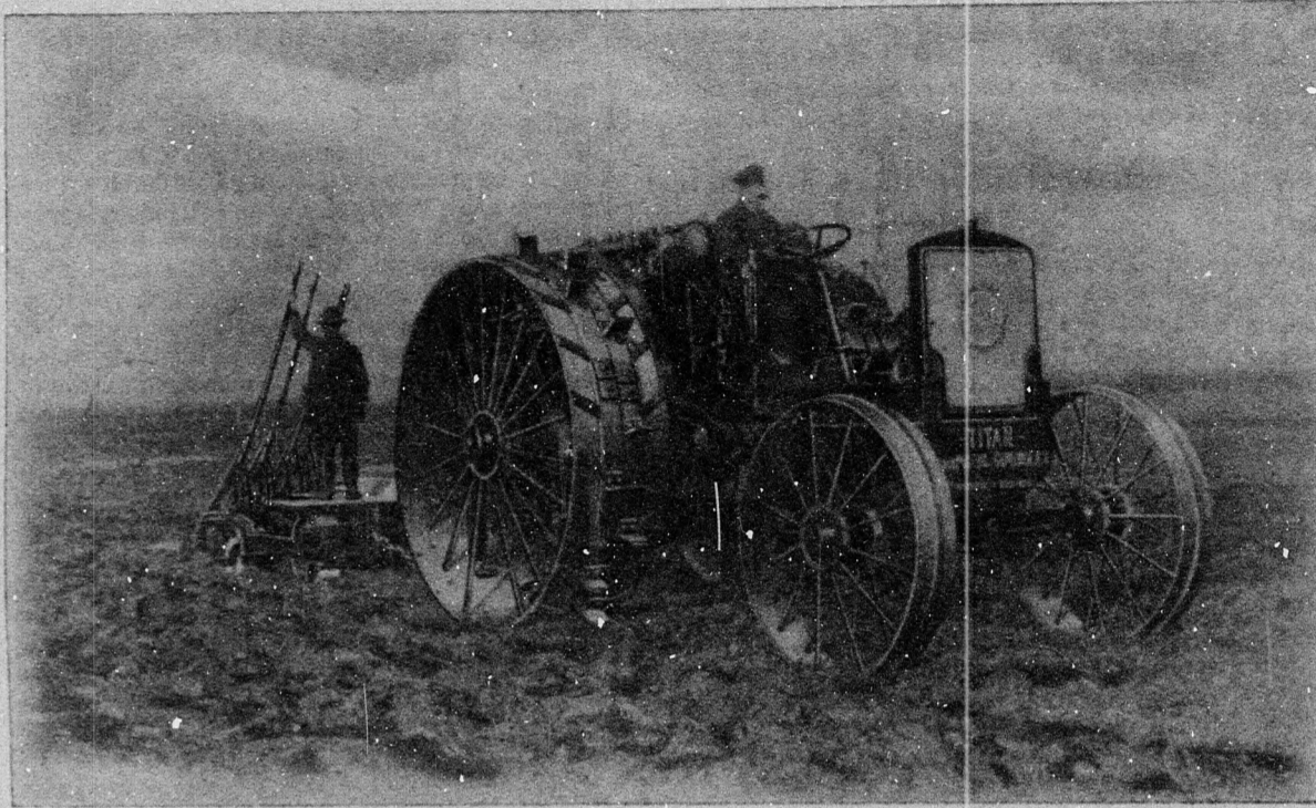
143. ábra. A szombathelyi Magyar Motor- és Gépgyár R.-T. „Titán” vontatós szántógépe.
