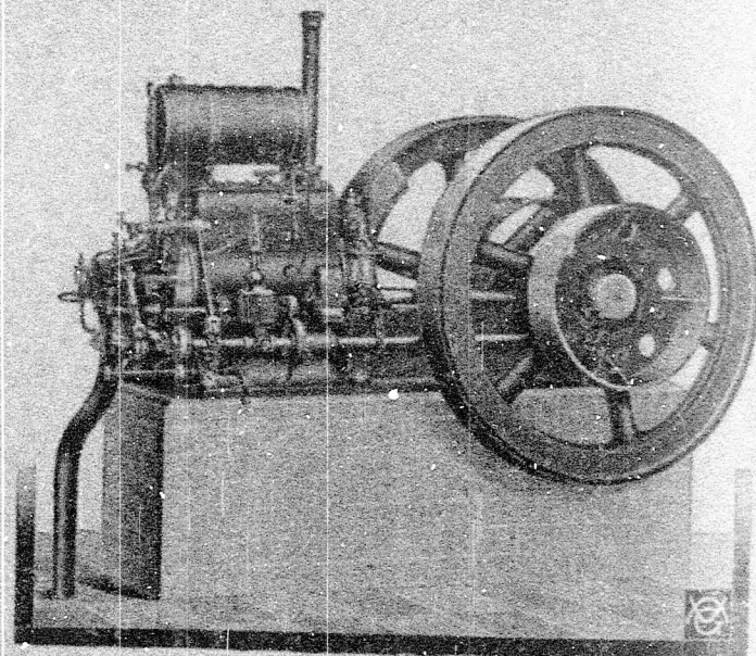
Legújabb rendszerű szab. stabil nyersolajmotor.
